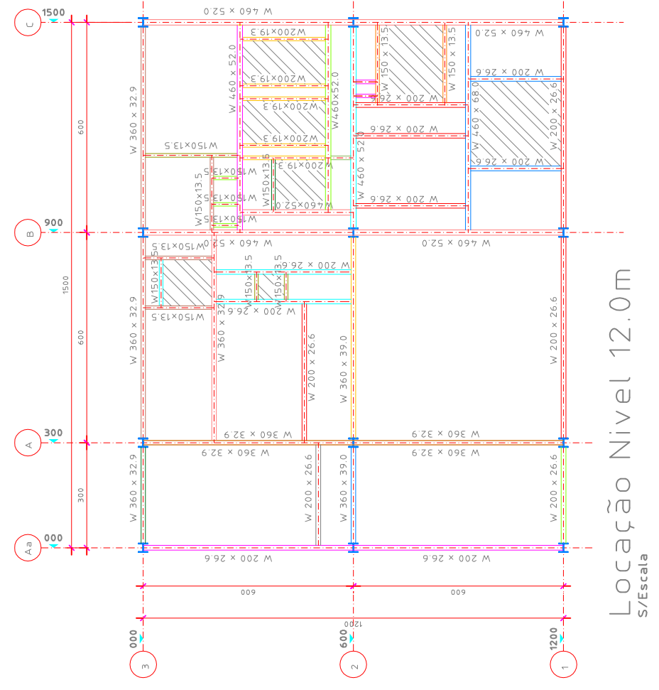
Locação Nivel 12.0m (Vigas Verticais) S/Escala
