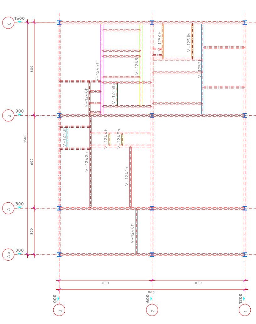
Locação Nivel 12.0m (Vigas Horizontais) S/Escala
