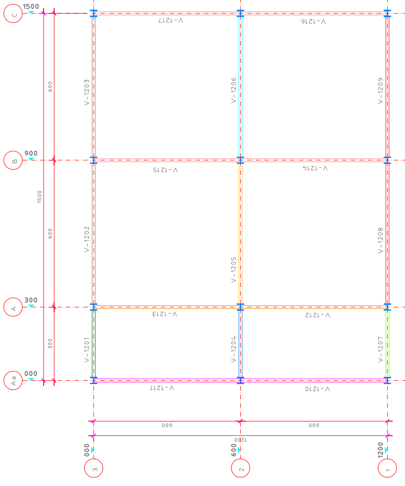
Locação Nivel 12.0m (Vigas Principais) S/Escala
