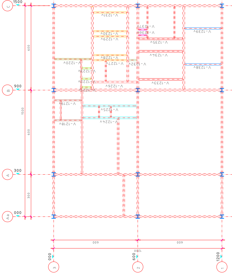
Locação Nivel 12.0m (Vigas Verticais) S/Escala
