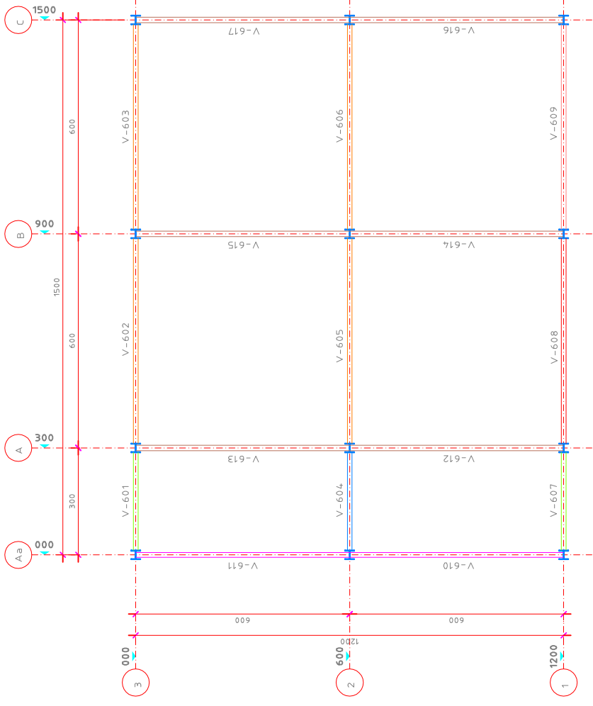
Locação Nivel 6.0m (Vigas Principais) S/Escala
