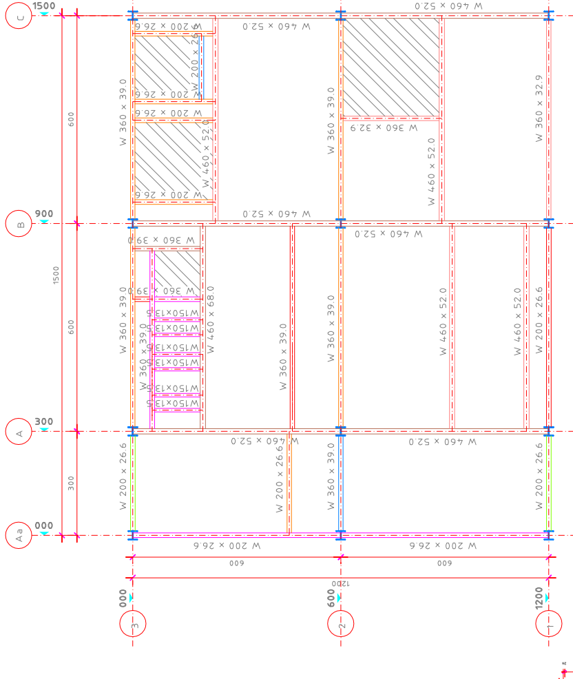
Locação Nivel 6.0m S/Escala
