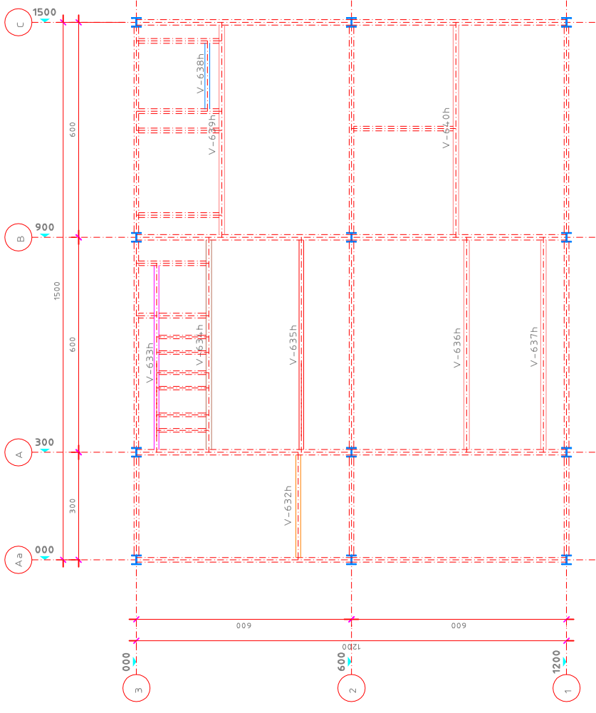
Locação Nivel 6.0m (Vigas Horizontais) S/Escala
