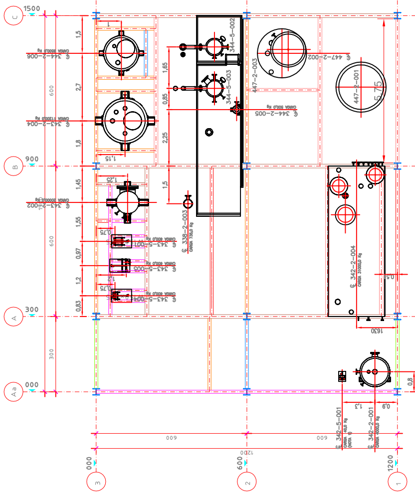
Locação Nivel 6.0m Com Equipamentos S/Escala
