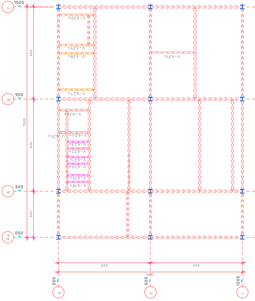
Locação Nivel 6.0m (Vigas Verticais) S/Escala
