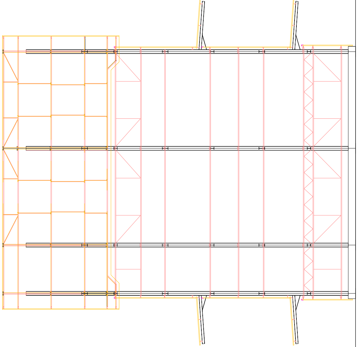
FACHADA LATERAL FECHAMENTO DETALHE TERÇAS S/ESCALA
