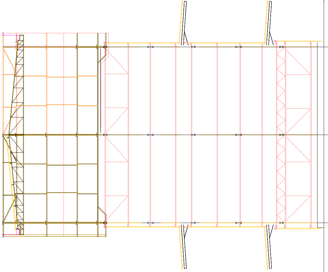
VISTA FRONTE FECHAMENTO DETALHES TERÇAS S/ESCALA
